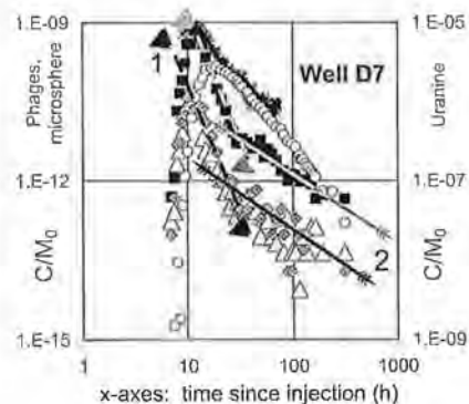
Fig. 4.20: Component concentration by well normalized to a) injectate concentration ( C/C_0 ) and b) injectate mass ( C/M_0 ) (log-log plot). Tracerkonzentration je Bohrung normalisiert auf a) Injektatkonzentration ( C/C_0 ) und b) Injektatmasse ( C/M_0 ) (log-log Plot).
