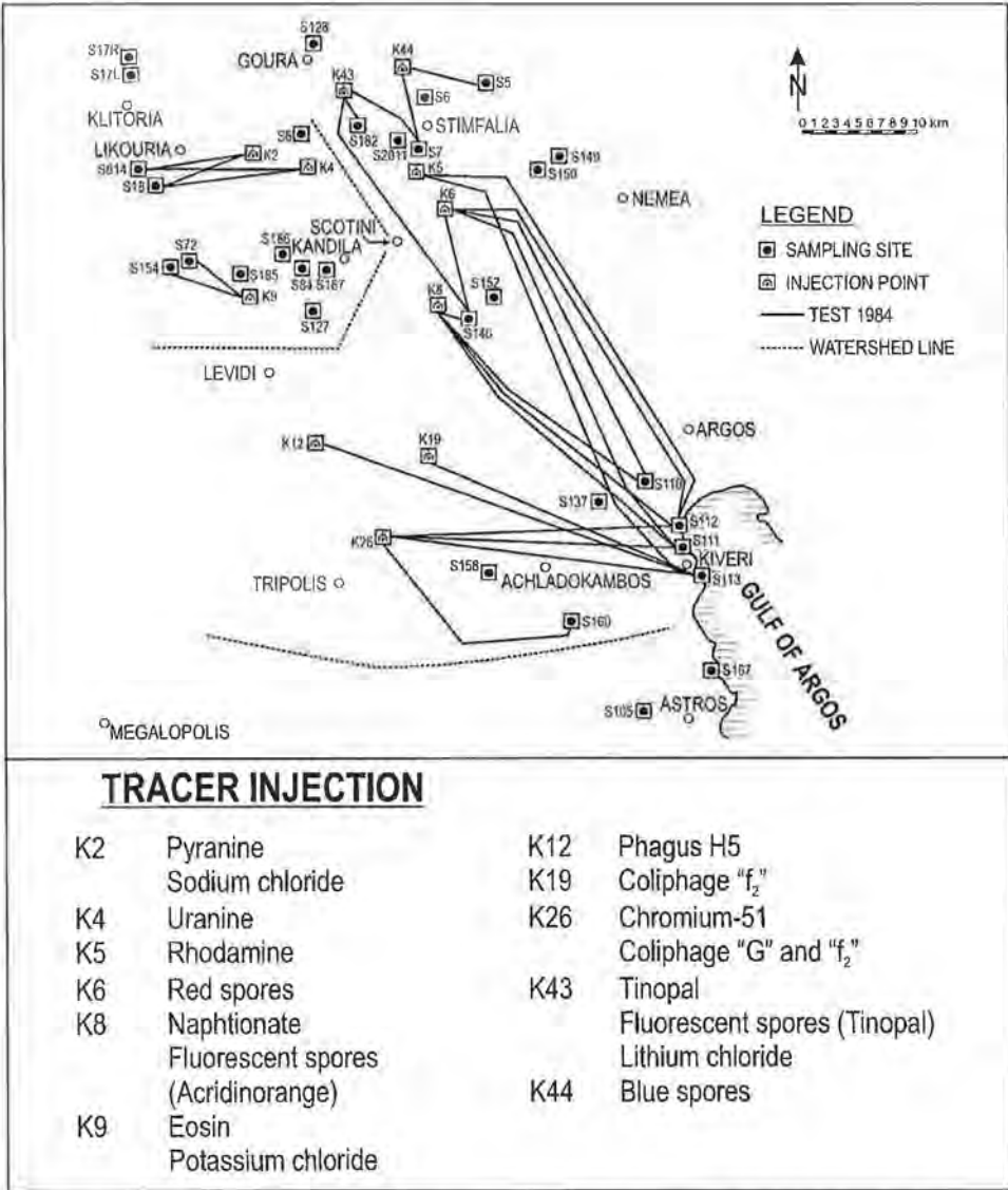
Fig. 2.3: Underground water connections between karst poljes (katastrothre) and springs in the investigation area of the Peloponnese, found by tracing tests with artificial tracers (from A. MORFIS & H. ZOJER, 1986). Im Markierungsversuch 1984 im Peloponnes zwischen Poljen und Quellen mit künstlichen Markierungen nachgewiesene Fließwege (aus A. MORFIS & H. ZOJER, 1986).
