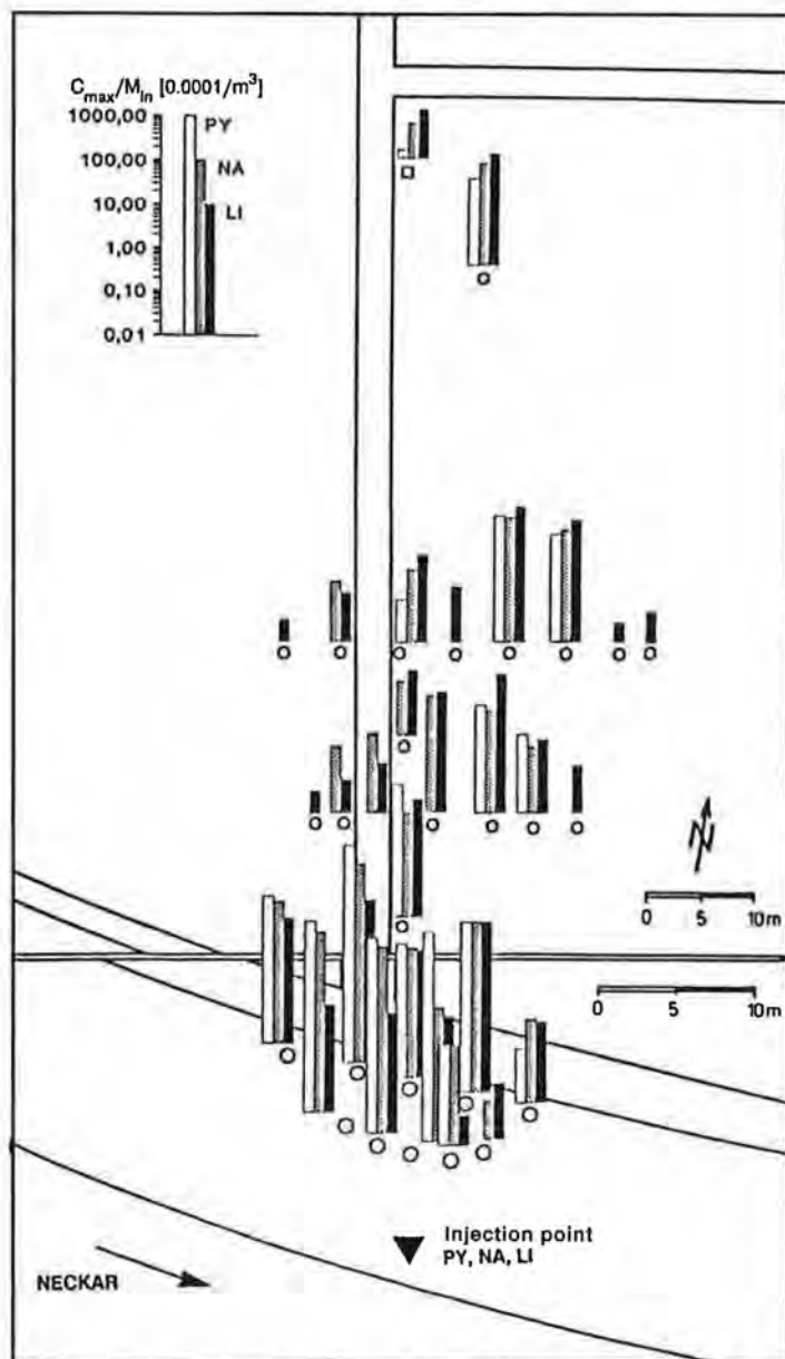
Fig. 1.2: Test site "Böckinger Wiesen", Heilbrom, Southwest Germany. Experimental well field in a 4 m thick confined gravel aquifer along an infiltration profile from the bank of river Neckar to a 100 m distant pumped well. The graph shows the result of a comparative tracer experiment with pyranine (PY), naphthionate (NA) and lithium (LI) (B. REICHERT, 1991). Testfeld „Böckinger Wiesen“, Heilbrom, Südwestdeutschland. Versuchsfeld in einem 4 m mächtigen, gespannten Kiesgrundwasserleiter entlang eines Infiltrationsprofils zwischen dem Neckar-Ufer und einem 100 m entfernt gelegenen Entnahmepumpen. Die Abbildung zeigt das Ergebnis eines vergleichenden Markierungsversuchs mit Pyranin (PY), Naphthionat (NA) und Lithium (LI) (B. REICHERT, 1991).
