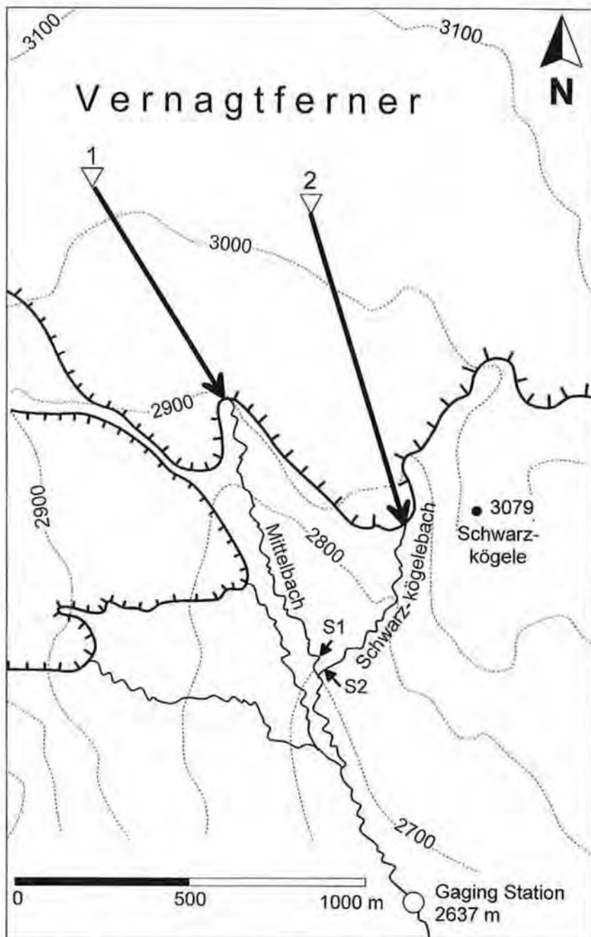
Fig. 3.2: Test area at Vernagt glacier. \nabla – injection points 1 and 2, \swarrow , \searrow – sampling points S_1 , S_2 , thick arrows – hypothetical subglacial water flows. Isohypes in metres above sea level. Kartenskizze des Untersuchungsgebietes auf dem Vernagtferner. \nabla – Einspeisestellen 1 und 2, \swarrow , \searrow – Beobachtungsstellen, dicke Pfeile – angenommene direkte Abflussbahnen der Markierstoffe.
