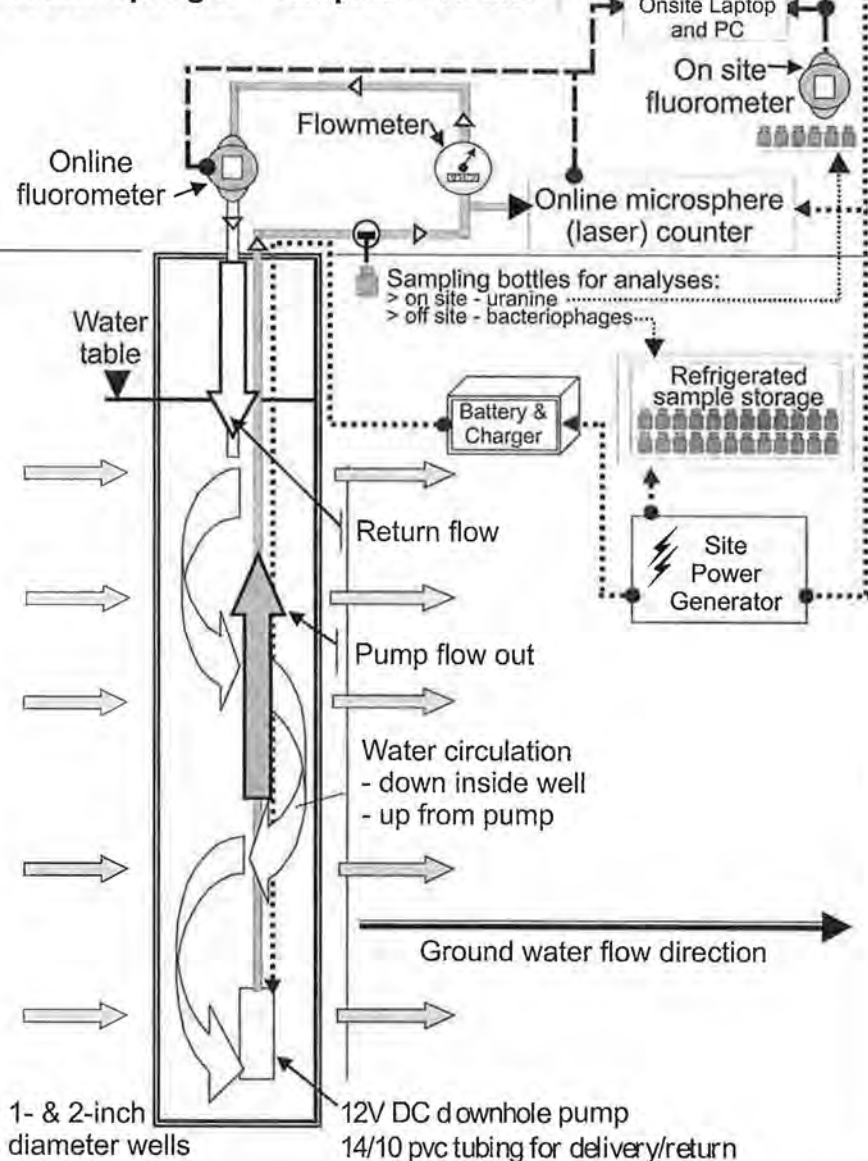
Fig. 4.11: Well equipment, sampling and on-site analysis instrumentation schematic diagram. Schematisches Diagramm: Bohrlochausrüstung, Probenentnahme- und in situ-Analysegeräte.
